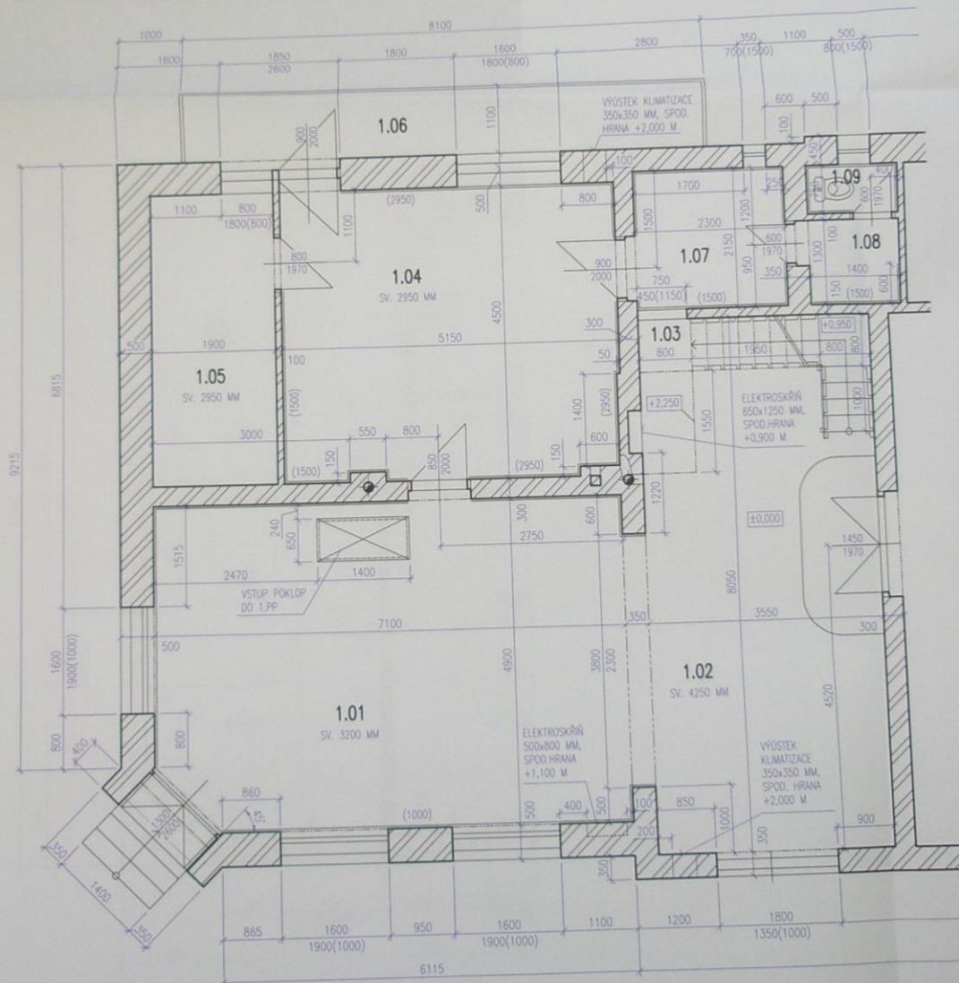
PŮDORYS 1.NP RESTAURACE SKALKA, M 1:50
