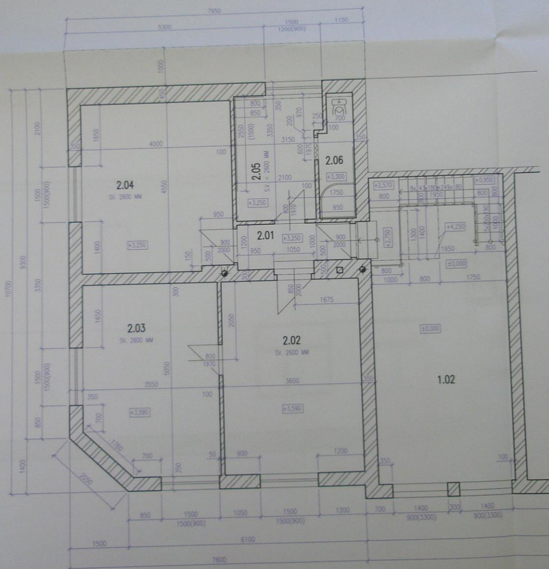
PŮDORYS 2.NP RESTAURACE SKALKA, M 1:50
